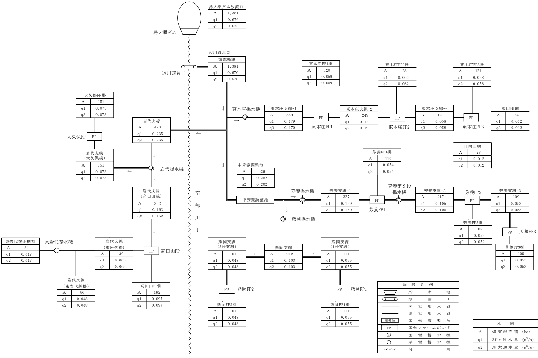
現況用水系統模式図
