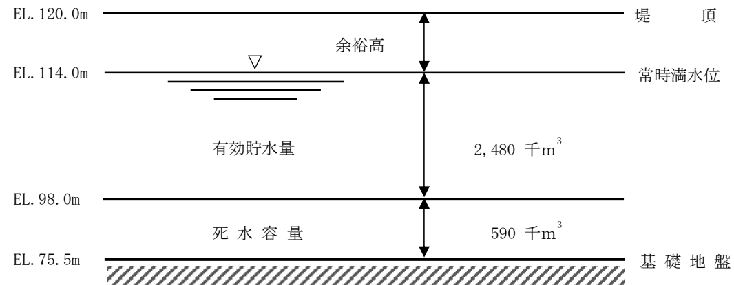
容量配分図
