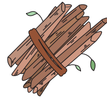
III 木くず
