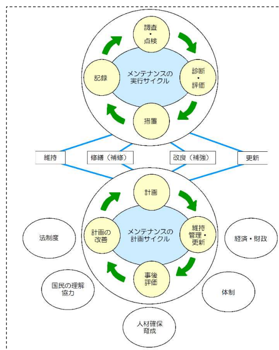
図2 メンテナンスサイクル ＜社会インフラメンテナンス学Ⅰ総論編Ⅱ工学編＞ 平成27年12月/公益社団法人土木学会
